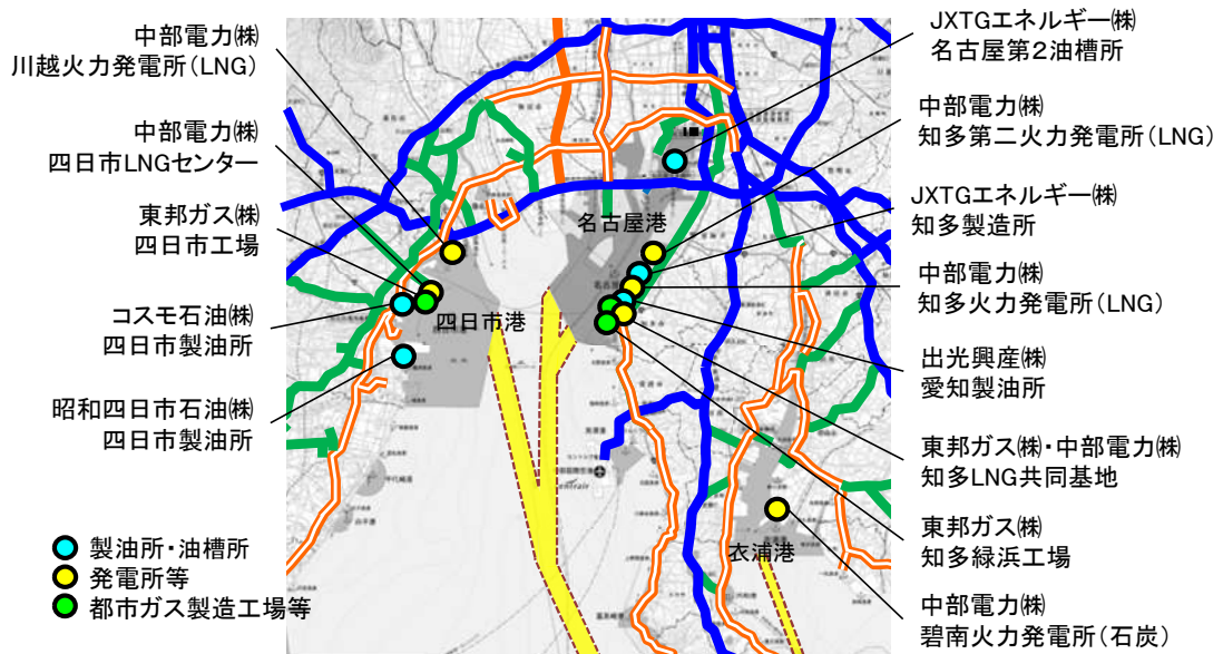
図 19 伊勢湾内の製油所・油槽所、発電所・都市ガス製造工場
