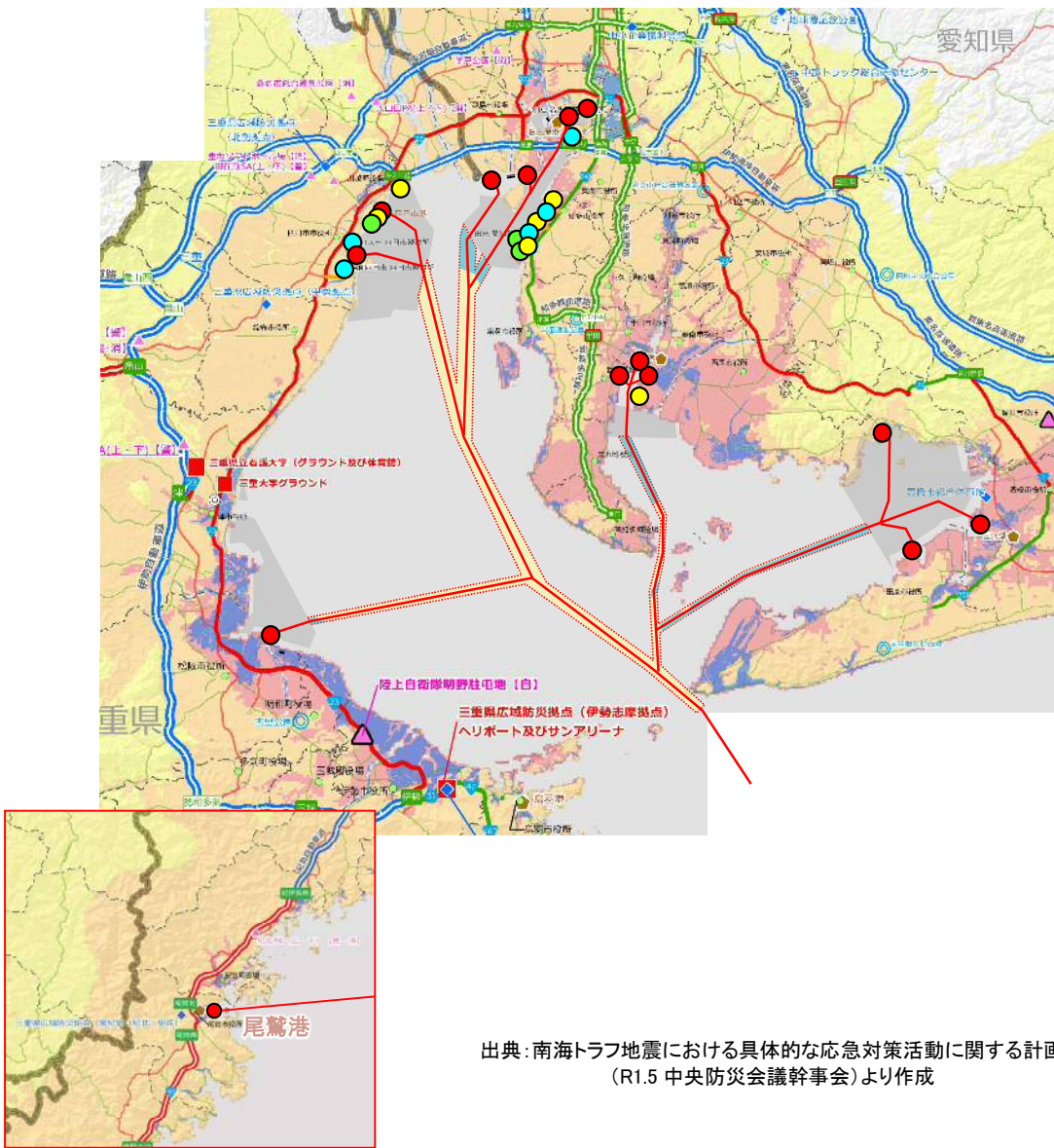
図 17 緊急確保航路等と南海トラフ地震の想定震度分布、防災拠点、緊急輸送路の重ね図
