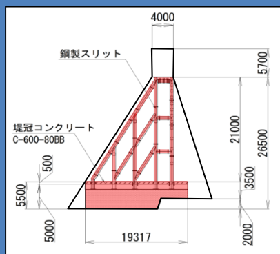
横断面図
