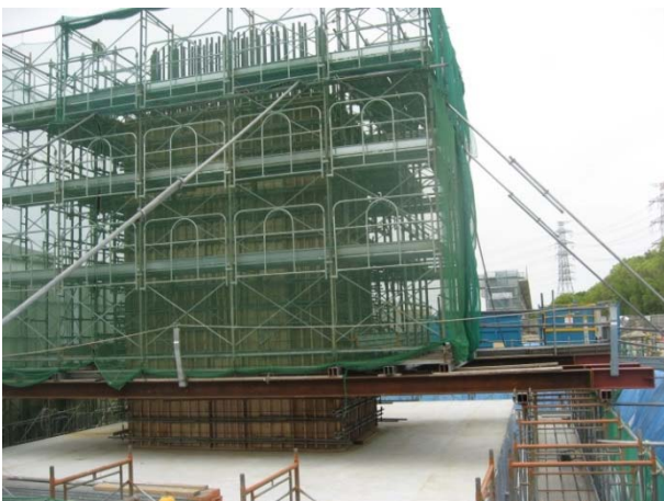
工事現場状況(5-2工区)・・・橋脚(コンクリート橋)
