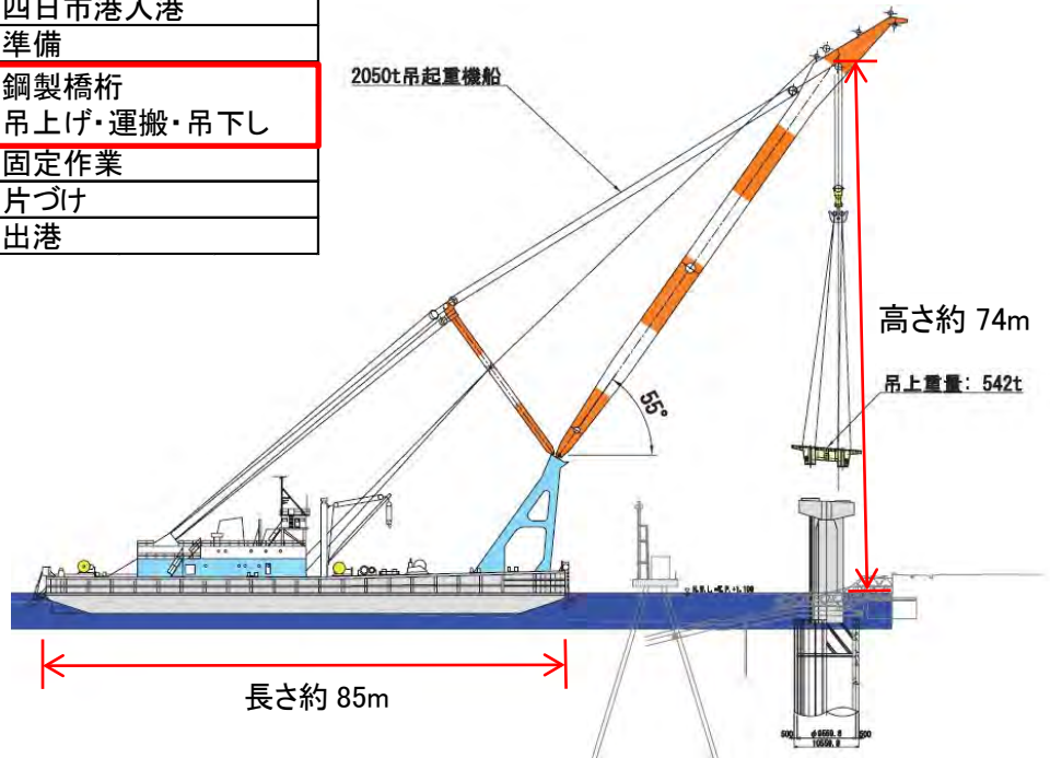
海上架設 イメージ図
