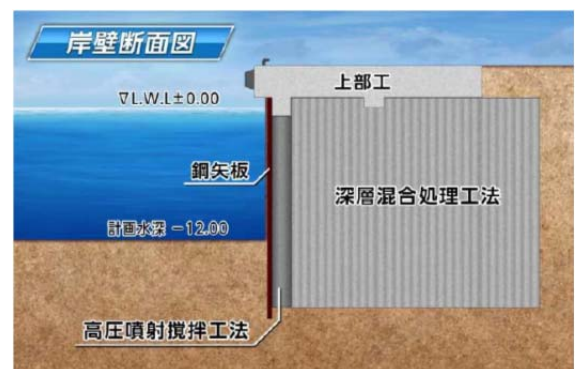
【耐震強化岸壁の断面図】
