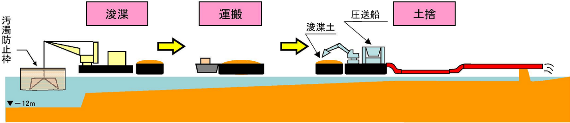
浚渫工事のイメージ
