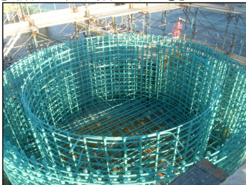
【(橋脚下部)鉄筋組立状況①】
