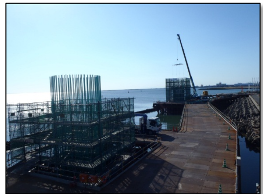
【(橋脚下部)鉄筋組立状況②】
