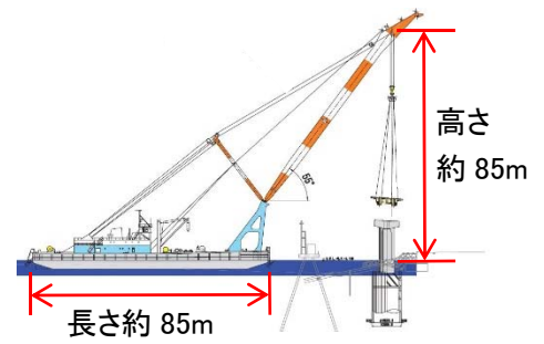
1,400t 吊 起重機船
