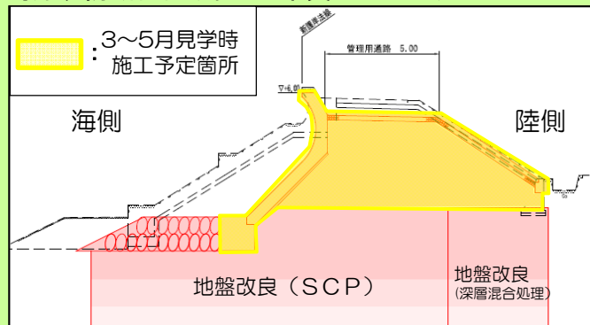
海岸堤防断面図（津地区栗真町屋工区）
