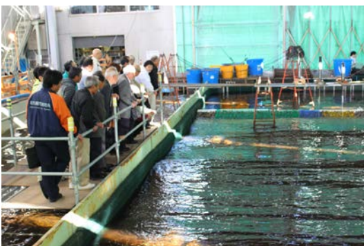
平面水槽で防波堤模型による消波効果を確認
